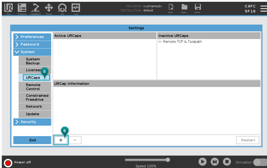
Abb. 3: Add URCap
