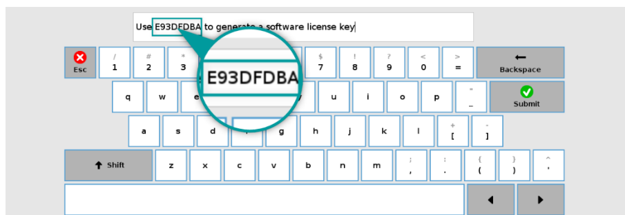
Abb. 9: Robot ID
